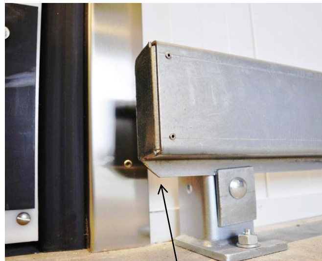
Avslut med ändplåt vid ev. pendeldörr med snedkapad skyddsbalk
